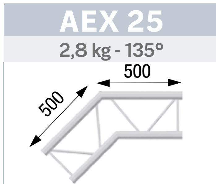
AL AEX25
